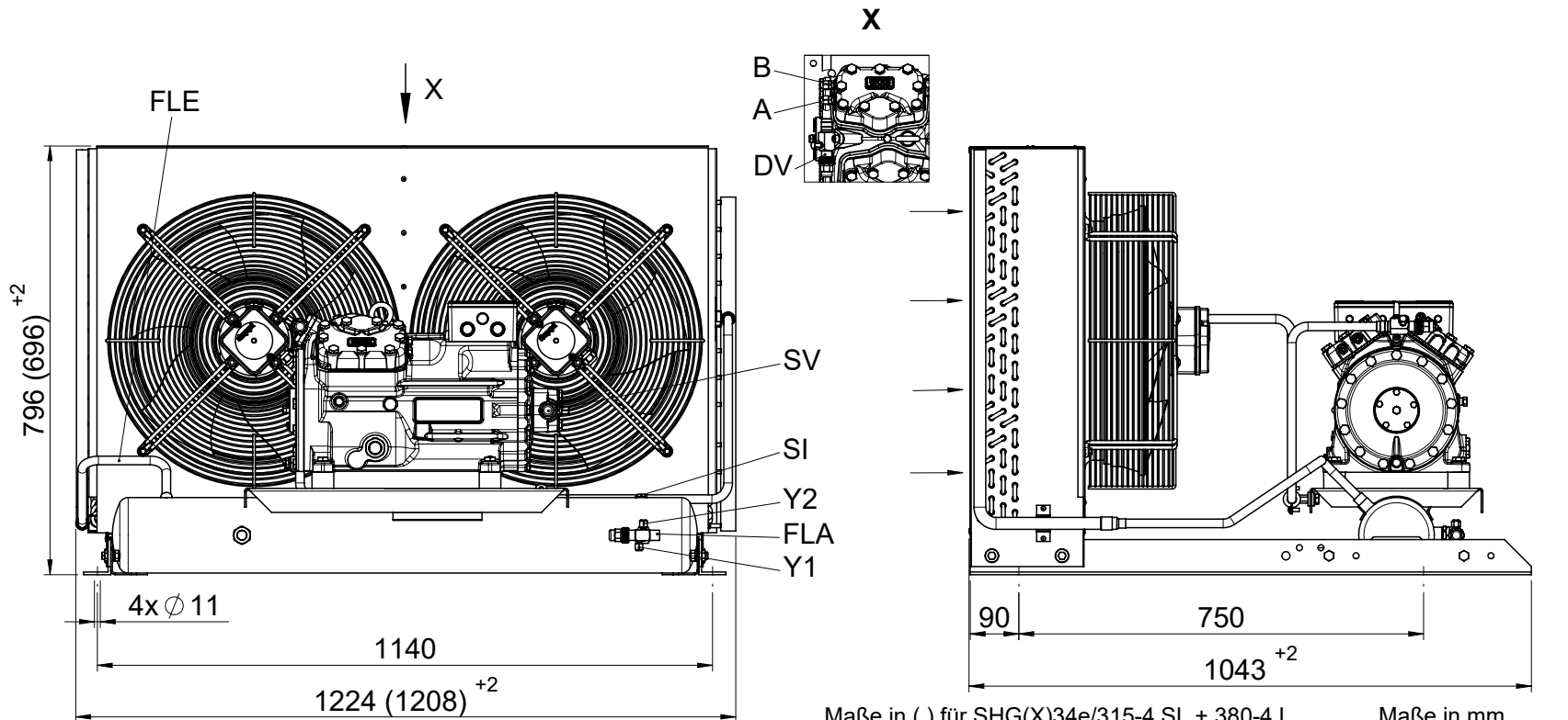
Maße in ( ) für SHG(X)34e/315-4 SL + 380-4 L Dimensions in ( ) for SHG(X)34e/315-4 SL + 380-4 L
